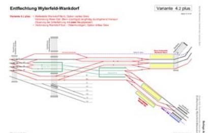
Studie Überwerfung Wylerfeld
